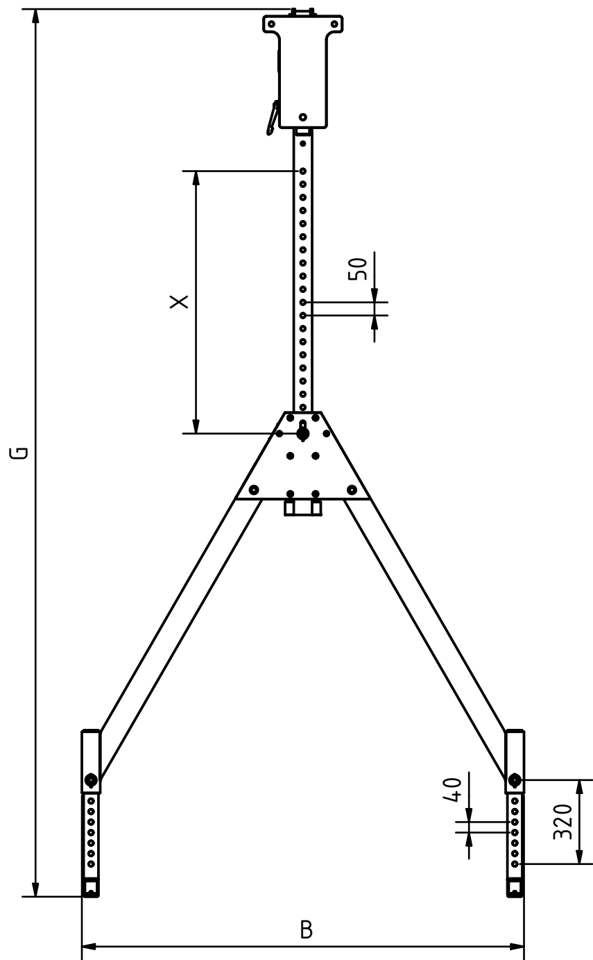
Abb. Kran Klappbar Modell Standard 4m Träger (112000-4) Maße in Millimeter (mm)
