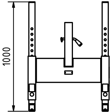
Seitengestell mit Steckaufnahme unterste Einstellung
