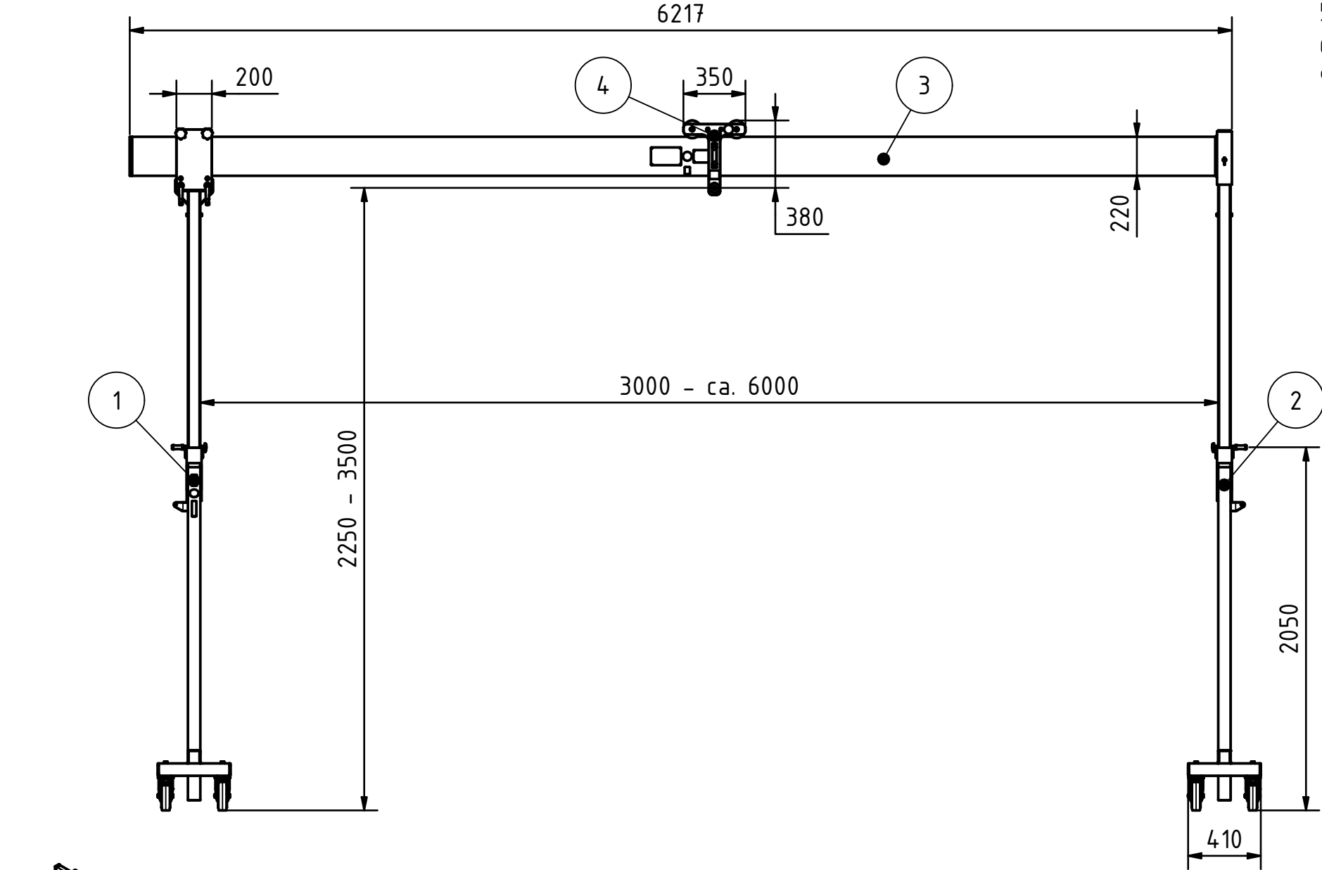
Seitengestell mit Steckaufnahme
