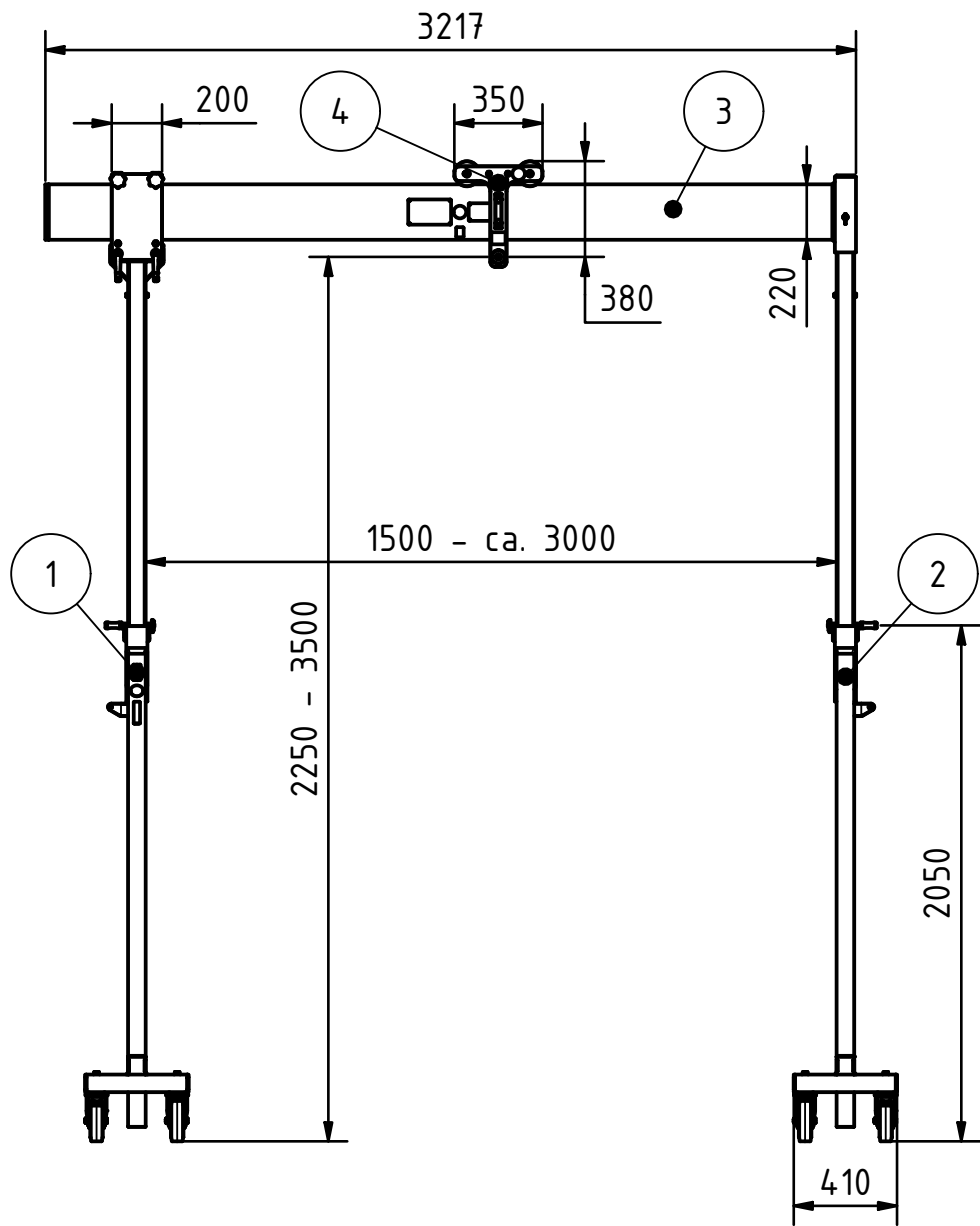
Seitengestell mit Steckaufnahme
