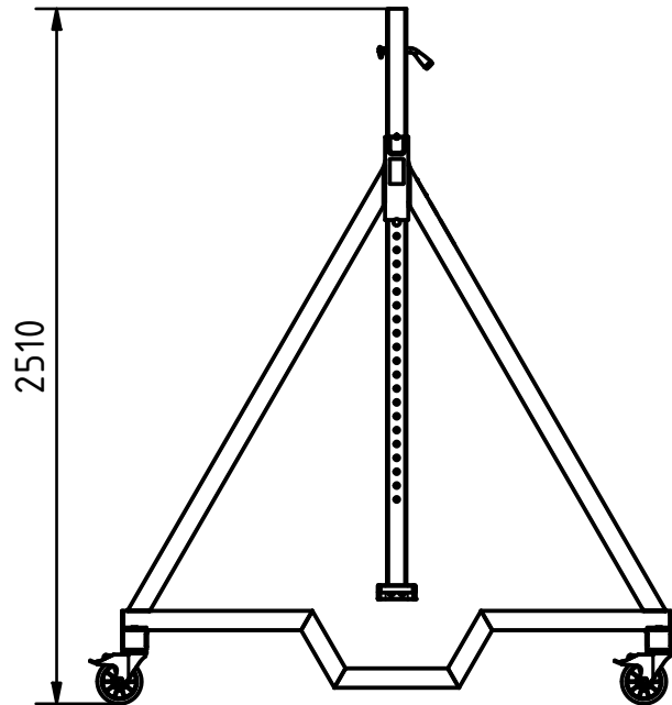
Seitengestell mit Steckaufnahme
