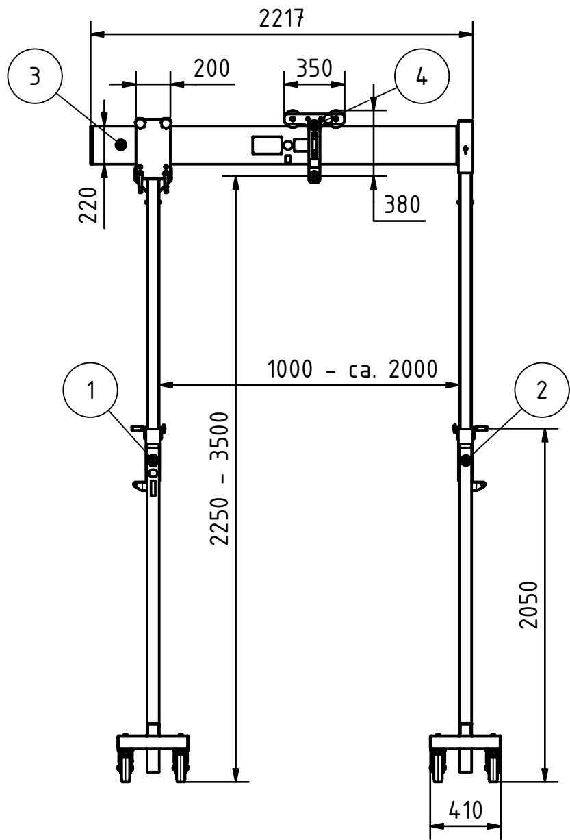
Seitengestell mit Steckaufnahme
