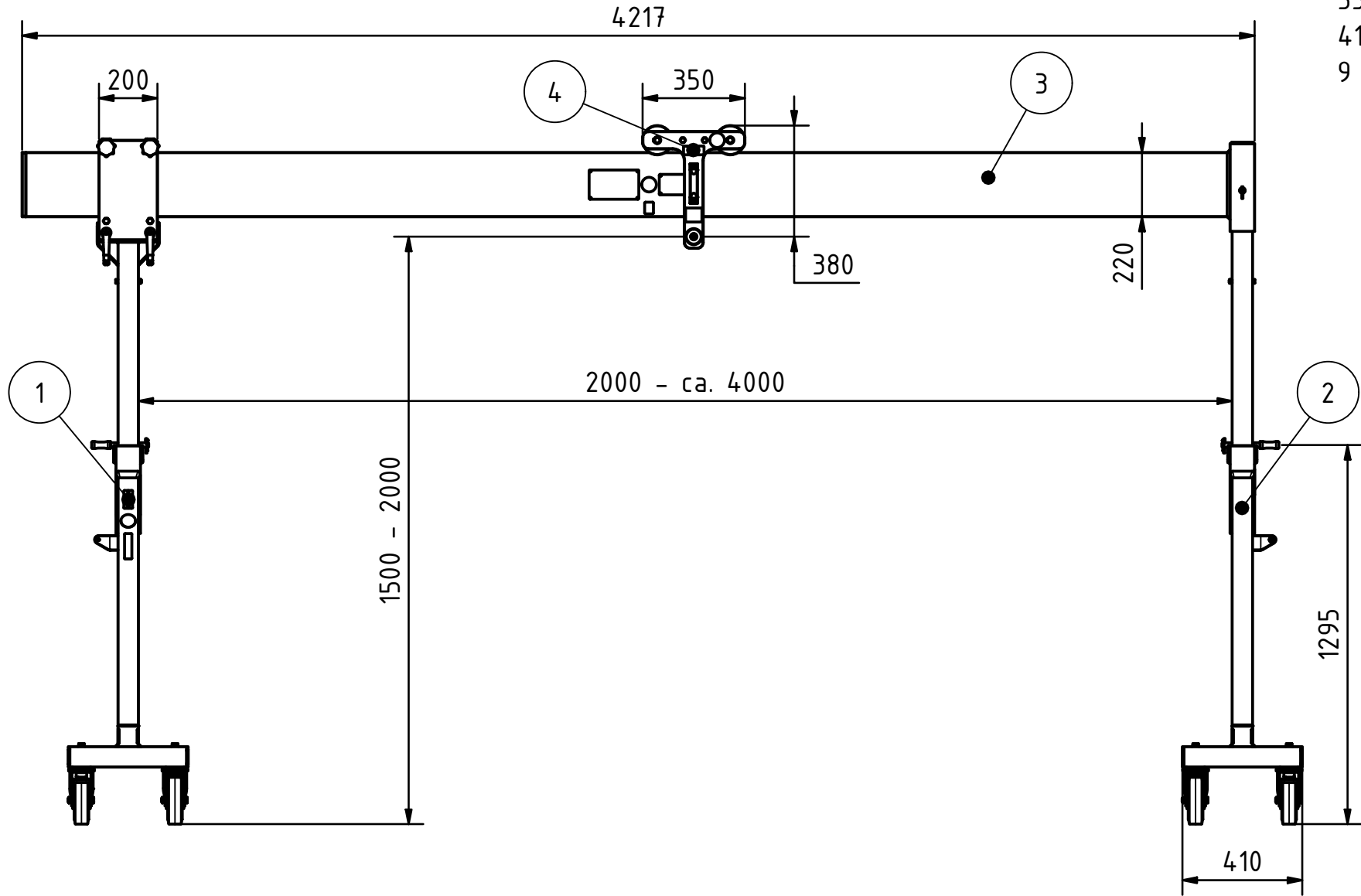
Seitengestell mit Steckaufnahme
