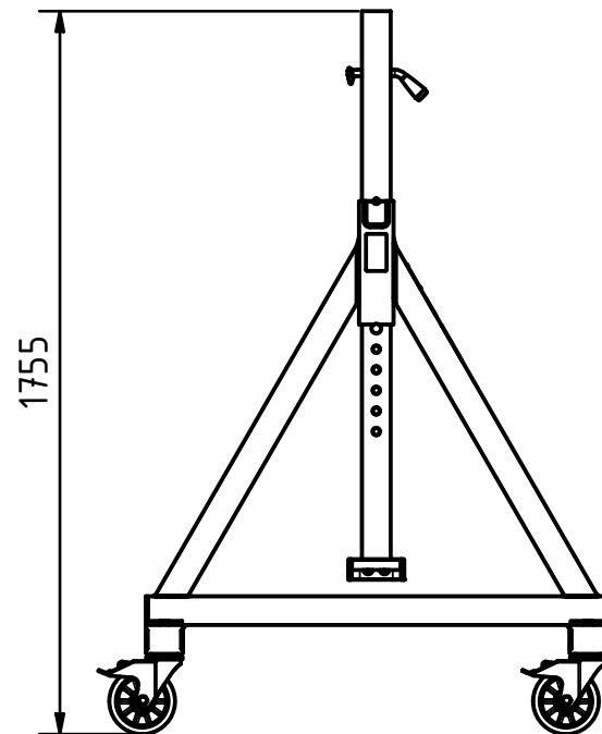
Seitengestell mit Steckaufnahme
