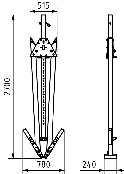
Seitengestell mit Steckaufnahme zusammengeklappt
