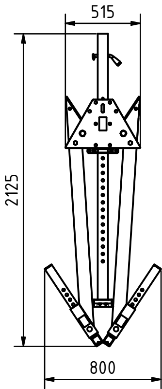
Seitengestell mit Steckaufnahme zusammengeklappt
