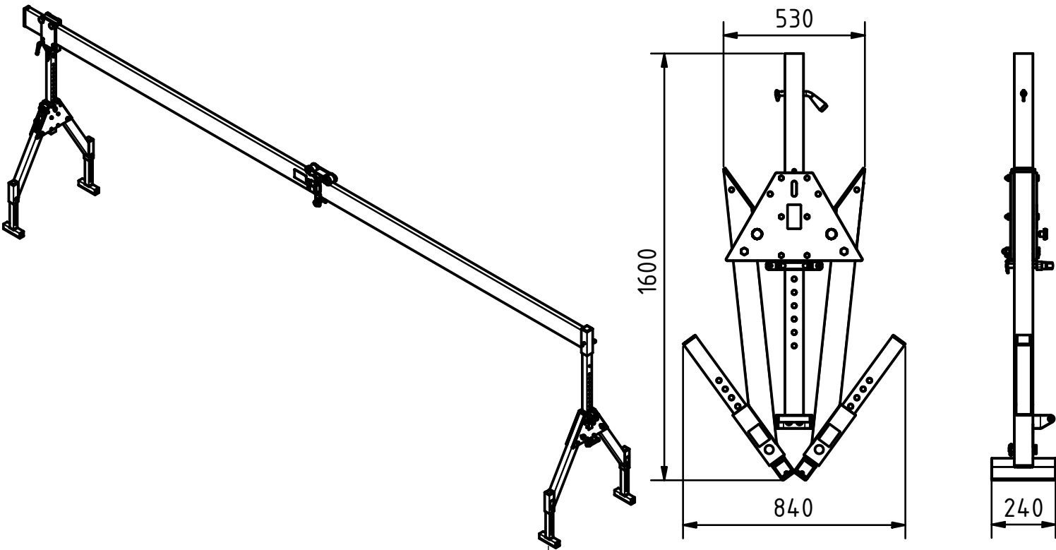
Seitengestell mit Steckaufnahme zusammengeklappt
