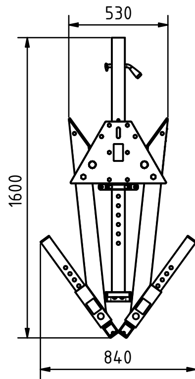
Seitengestell mit Steckaufnahme zusammengeklappt
