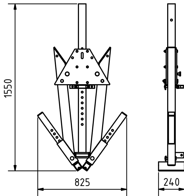
Seitengestell ohne Horizontalversteller zusammengeklappt
